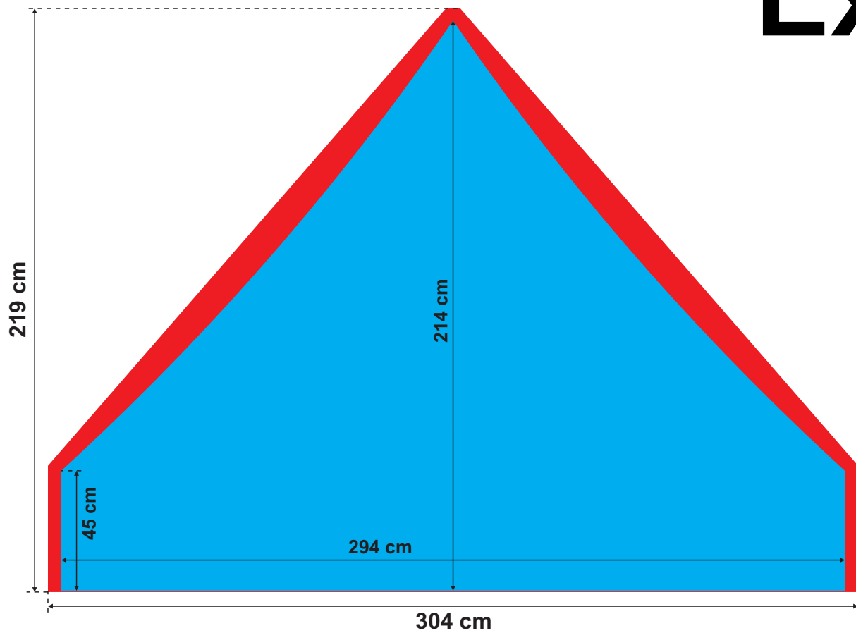
OBERTEIL ( x4 )
