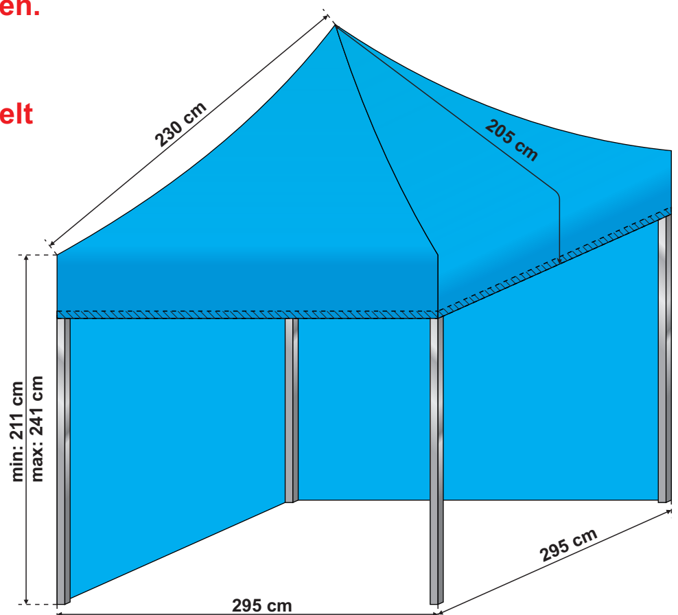
SEITENWAND ( x4 )
